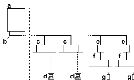
a Наружный блок системы VRV IV-S на основе теплового насоса
