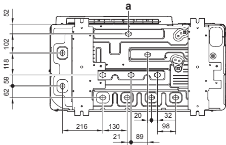
а Сливные отверстия
