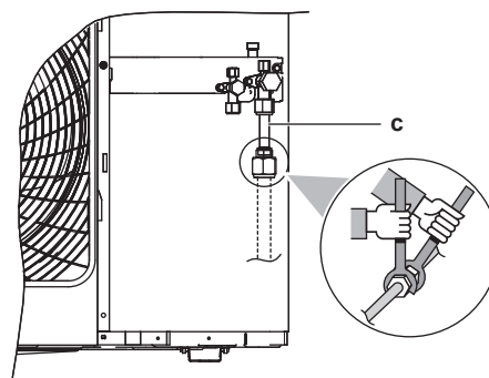
с Вспомогательный патрубок трубопровода газообразного хладагента (только модель RXYSCQ6)
